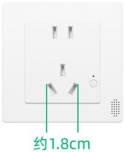
86型 10A智能墙壁插座 S2 GSPW1B2
