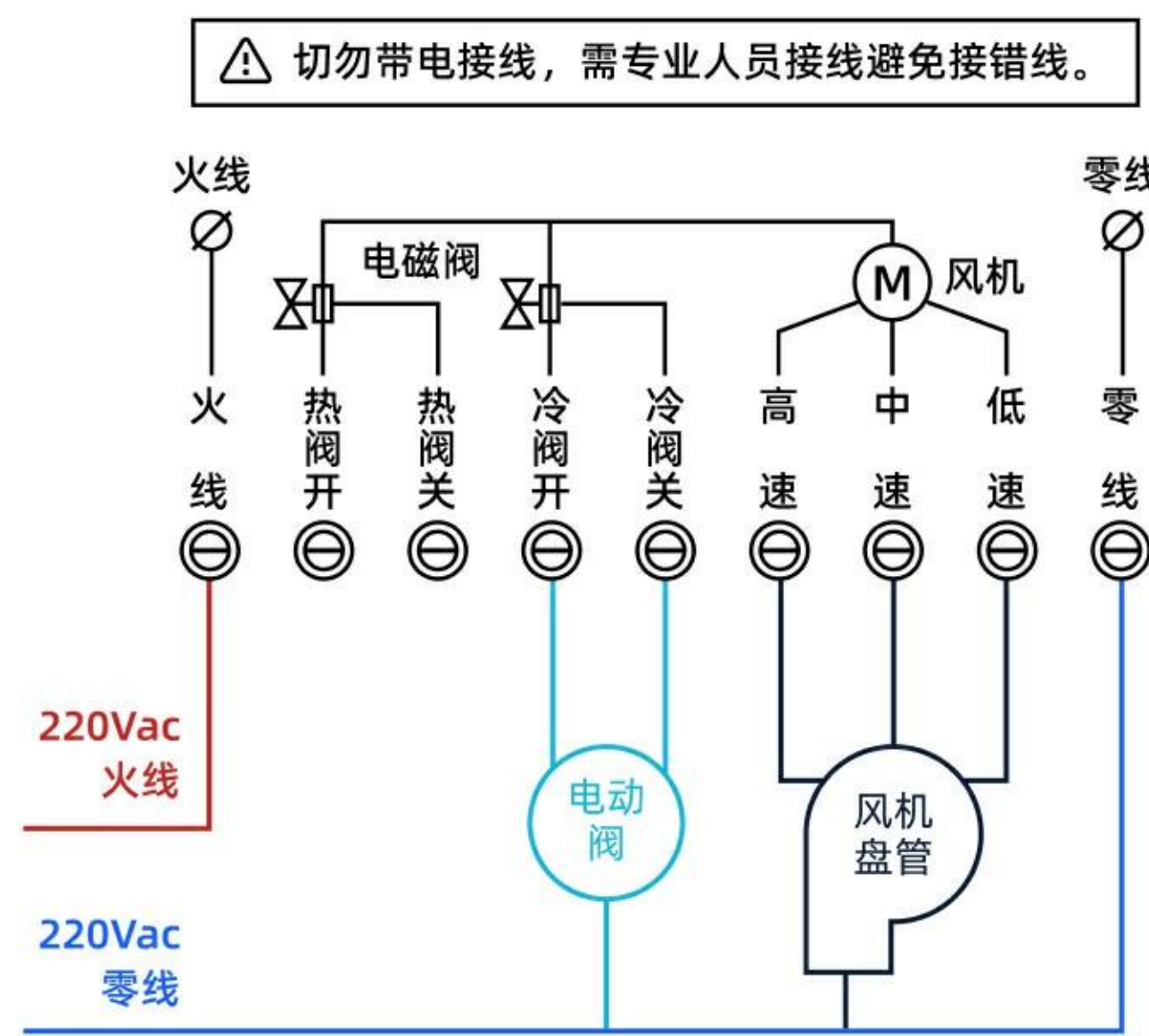
三管制空调智能控制面板-Wifi版 GSKWWD4B
