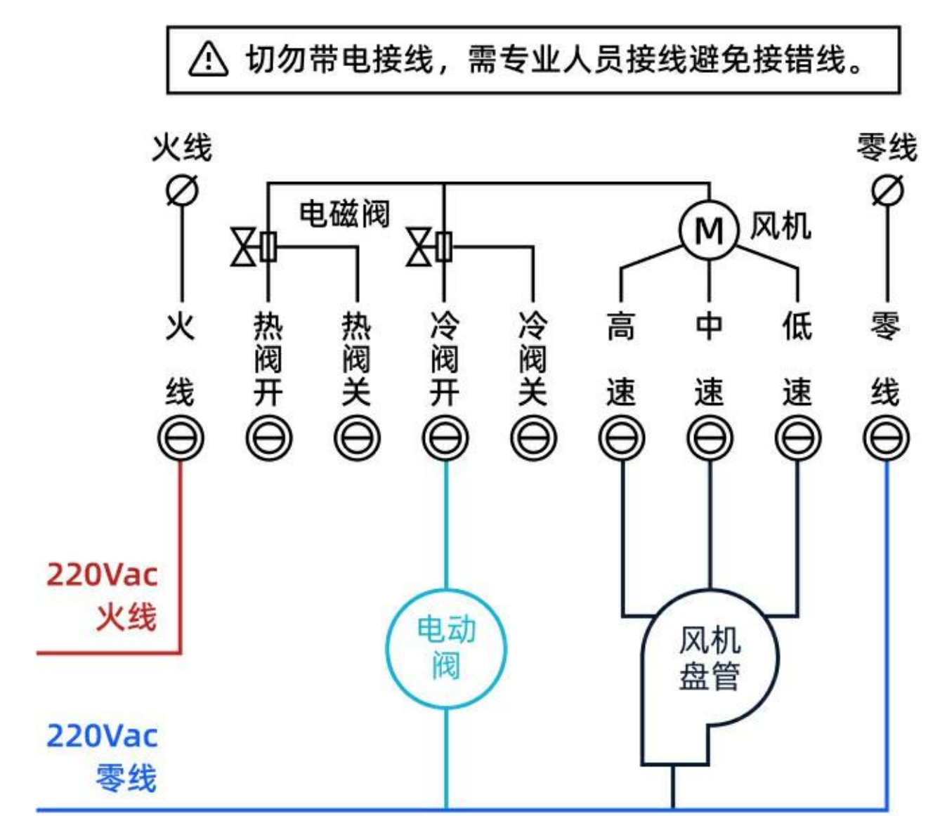
二管制空调控制面板-Wifi版 GSKWFD5B
